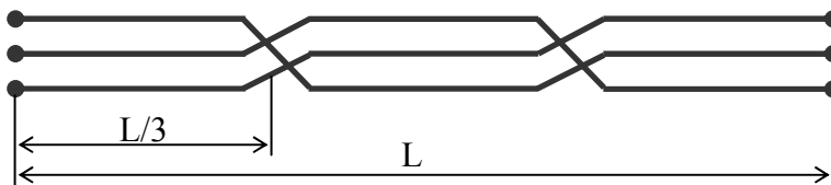
Рисунок 2.17 – Транспозиция кабелей
