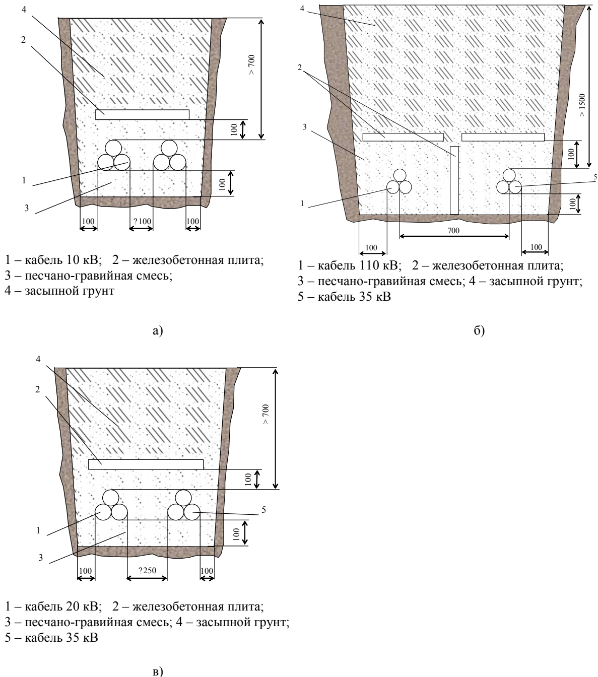
Рисунок 3.3 – Примеры прокладки кабелей в траншее
