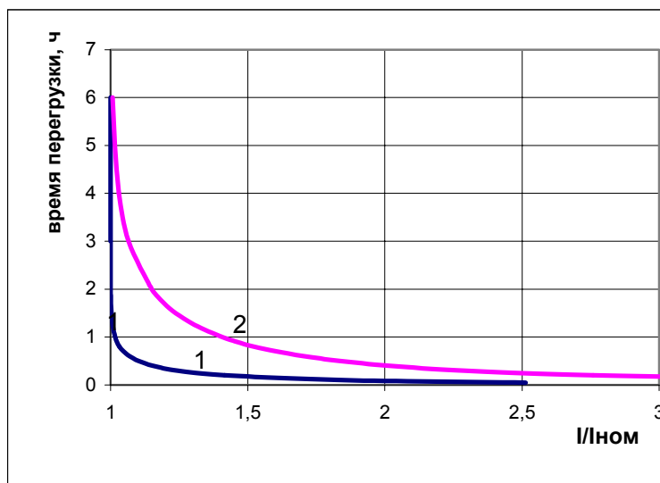
Рисунок 2.11 – Перегрузочная кривая при первоначальном включении одножильного кабеля:
