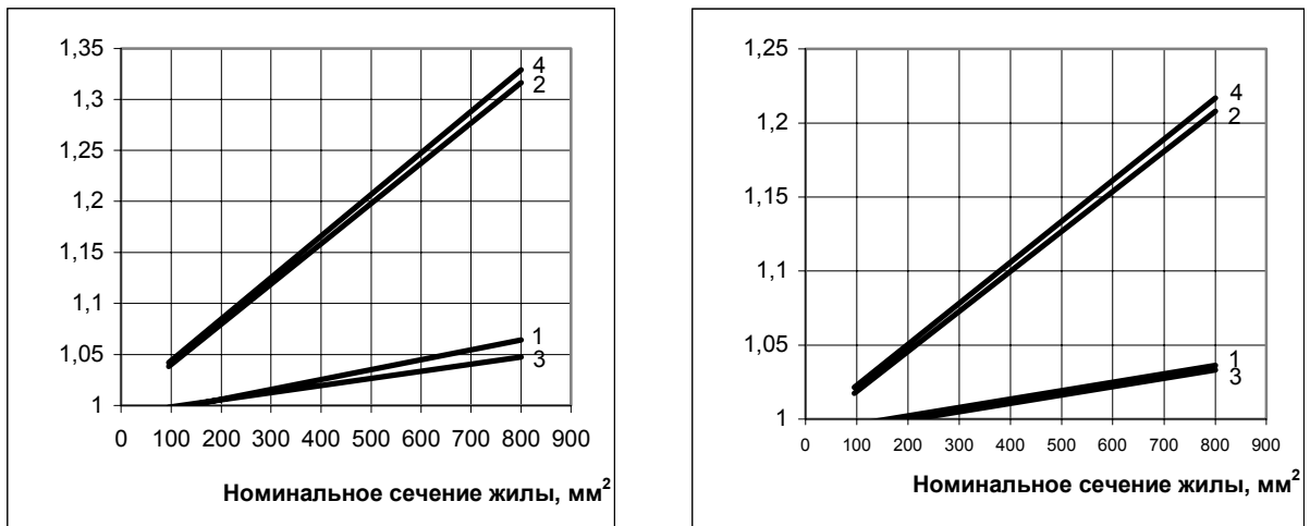
а) б) 1 – кабели проложены в земле треугольником; 2 – кабели проложены в воздухе треугольником; 3 – кабели проложены в земле в плоскости; 4 – кабели проложены в воздухе в плоскости
