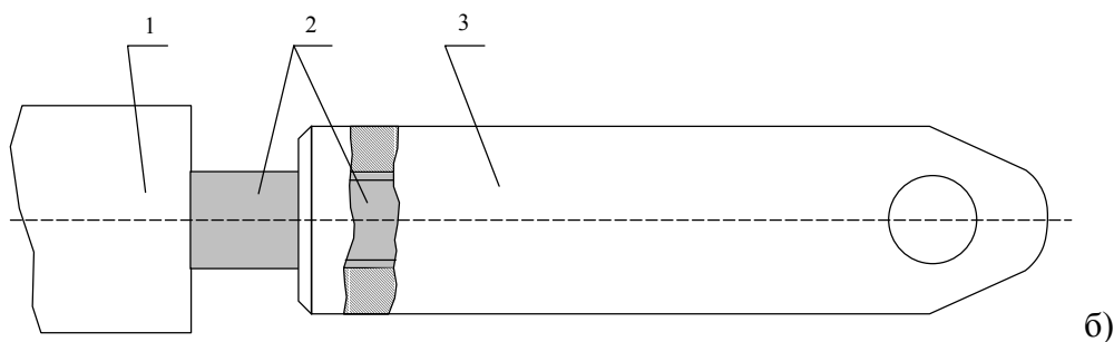
1 – кабель; 2 – жила кабеля; 3 – приспособление для тяжения
