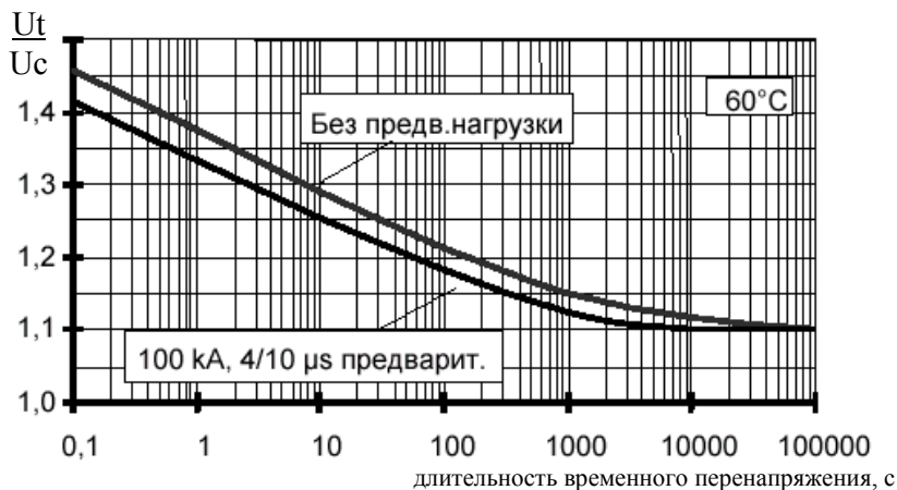
U_t – максимальное напряжение, которое прикладывается к выводам ОПН в случае замыкания на землю (временное перенапряжение), кВ; U_c – рабочее напряжение ОПН, кВ
