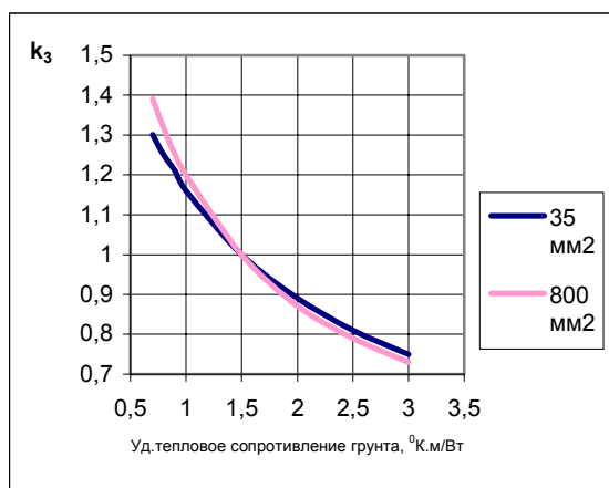
Рисунок 2.3 – Поправочные коэффициенты k_3 для удельных тепловых сопротивлений грунта, иных, чем 1,5 К·м/Вт, для одножильных кабелей, проложенных непосредственно в грунте
