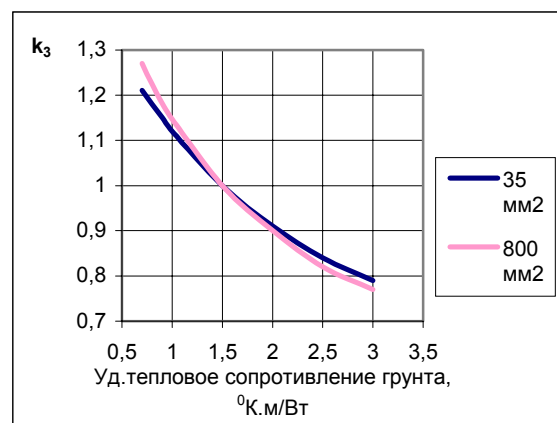
Рисунок 2.4 – Поправочные коэффициенты k_3 для удельных тепловых сопротивлений грунта, иных, чем 1,5 К·м/Вт, одножильных кабелей в трубах, проложенных в грунте
