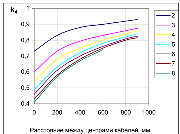
Рисунок 2.8 – Поправочные коэффициенты k_4 для групп трехфазных цепей одножильных кабелей, проложенных непосредственно в грунте
