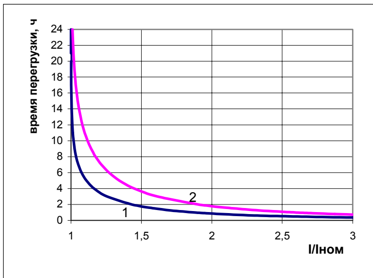
Рисунок 2.12 – Перегрузочная кривая при первоначальном включении трехжильного кабеля:
